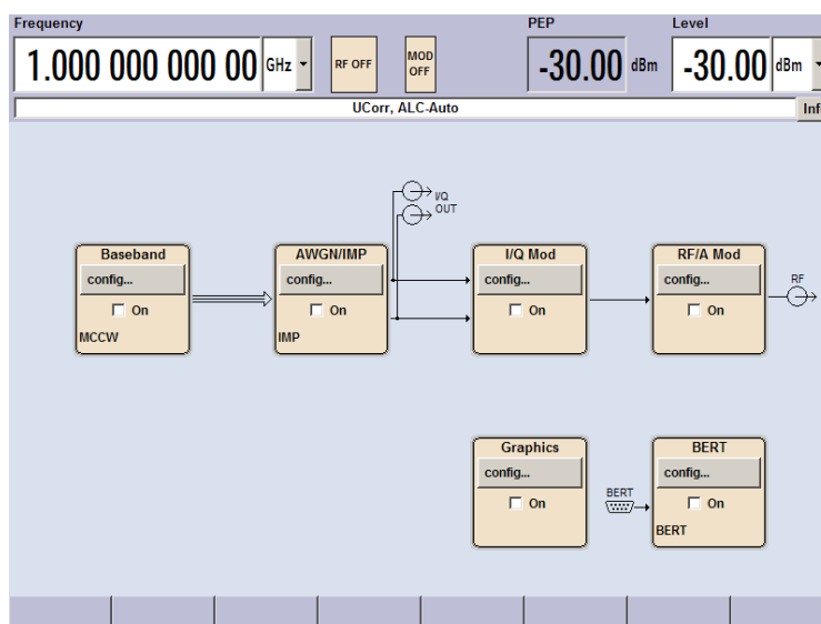
図 4-1: すべての機能を装備した R&S SMJ のブロック・ダイアグラム
