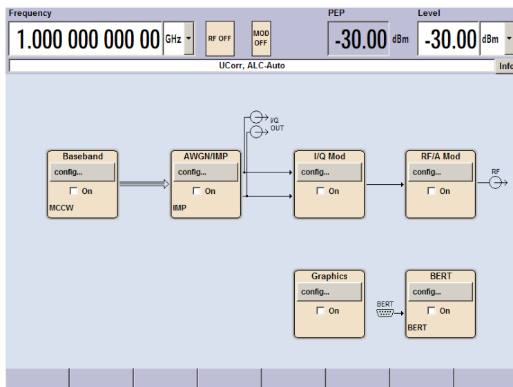
図 3-1: すべての機能を装備した R&S SMJ のブロック・ダイアグラム
